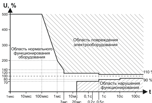
Рис. 1. Кривая работы электрооборудования ITIC (CBEMA). ( http://www.home.agilent.com/upload/cmc_upload/All/1_1.pdf?&cc=UA&lc=eng ).
